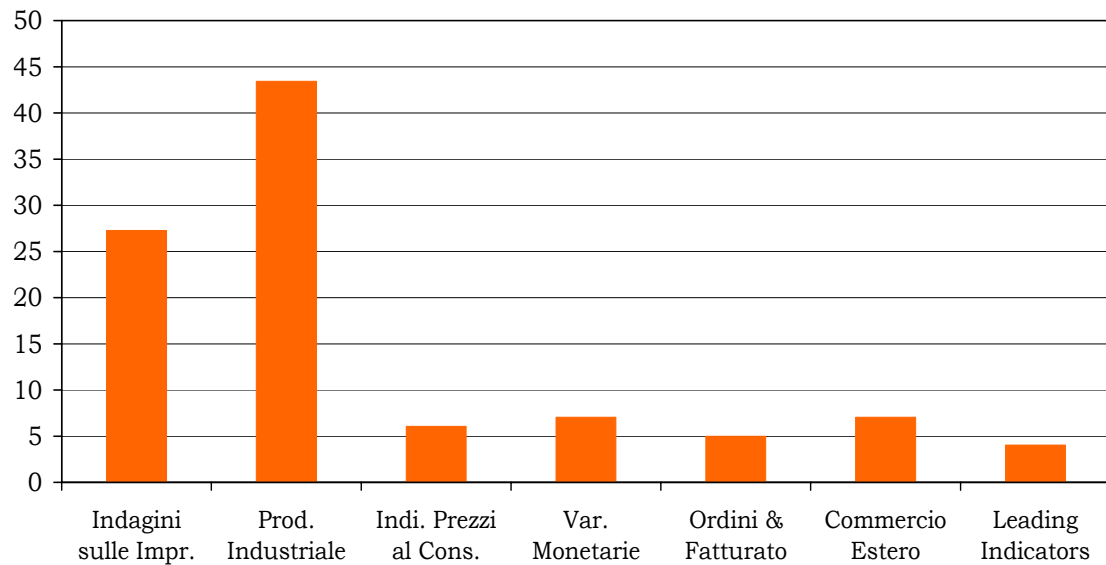
Grafico 2 - Determinanti per la stima dell'indicatore CoinCer per il mese di novembre 2013
